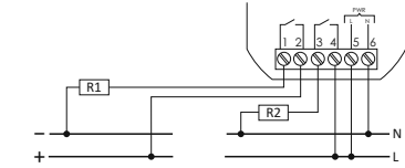
R1: Różne napięcia zasilania dla przełącznika i odbiornika
